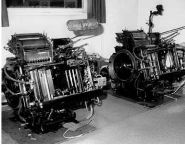
Stanzmaschine für die ursprüngliche Buchstabenproduktion
